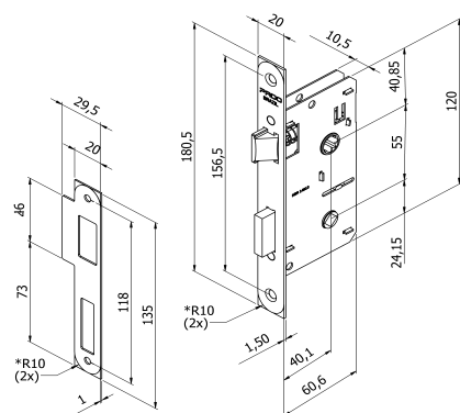
Máquina 40CB c/ Contra Testa * Versão Raio
