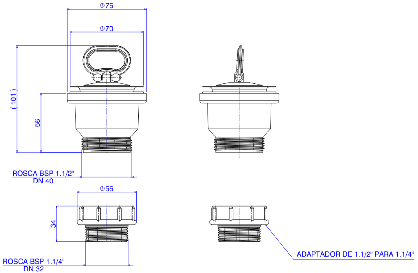
Desenho Técnico
